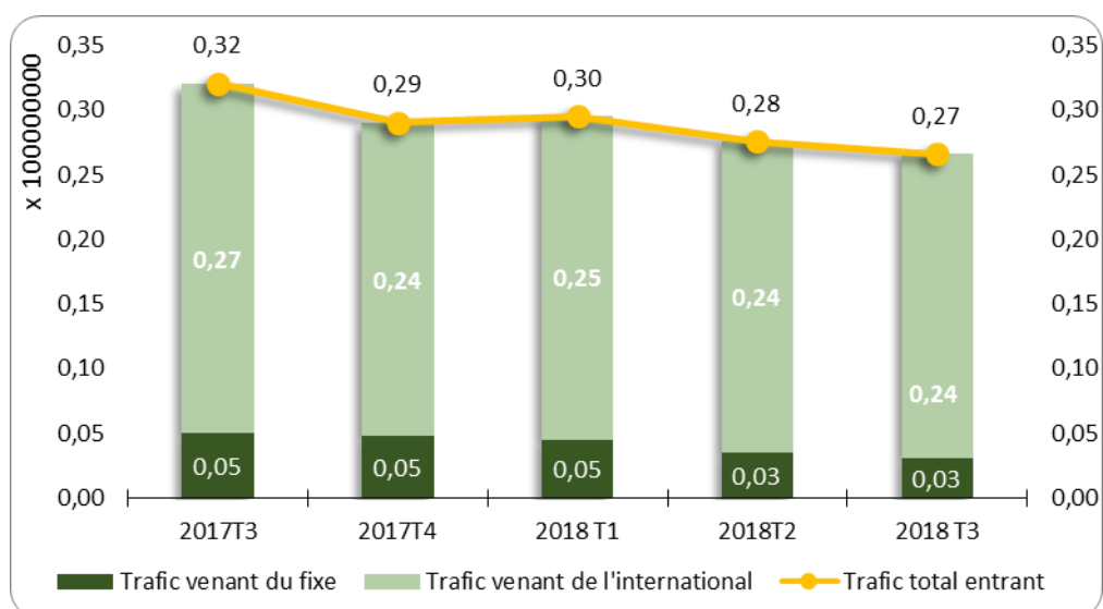
Graphique 12 : Evolution du trafic mobile entrant
