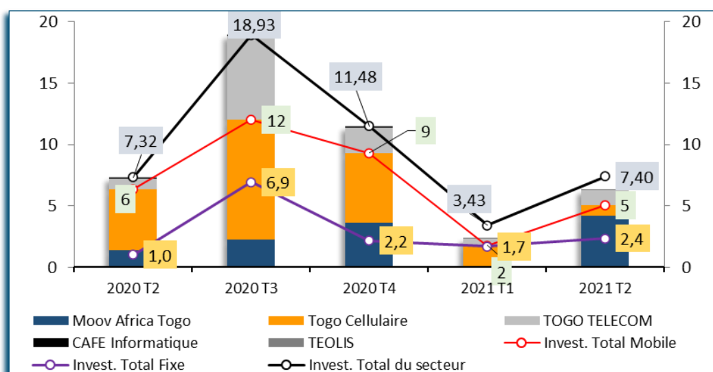
Graphique 18 : Evolution de l'investissement par opérateur (en milliard de Fcfa)
