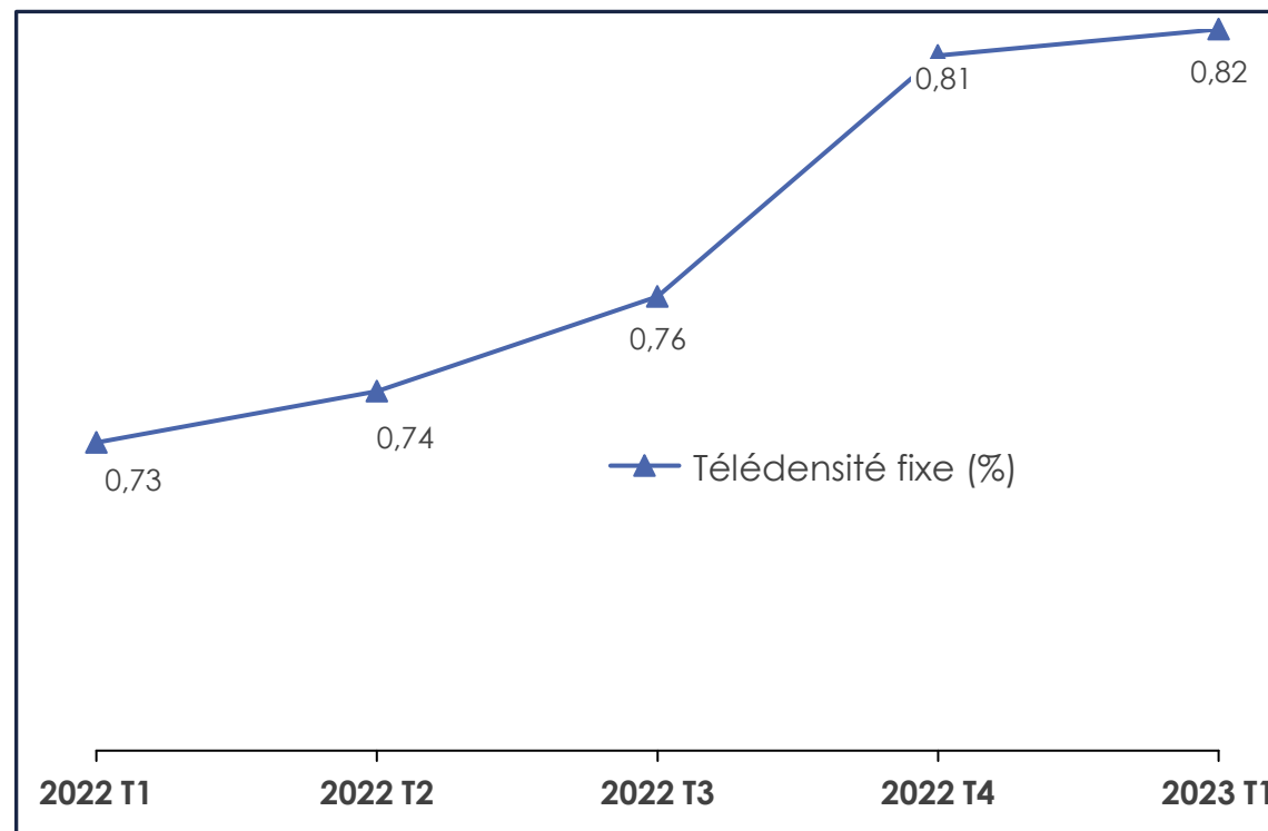
Télédensité fixe (%)
