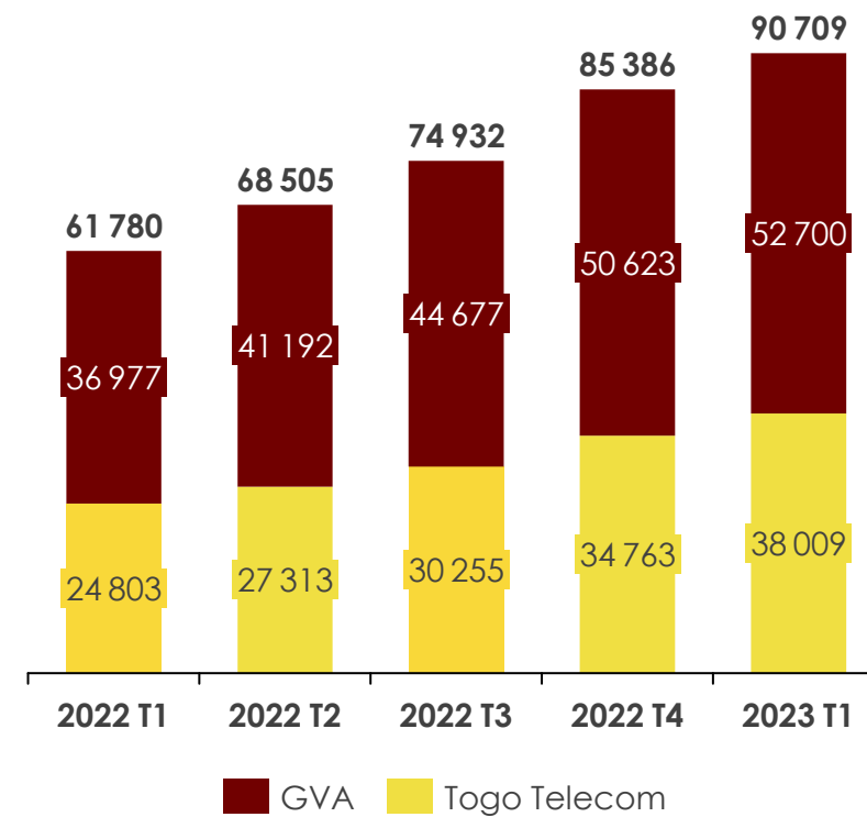
Abonnés FTTH
