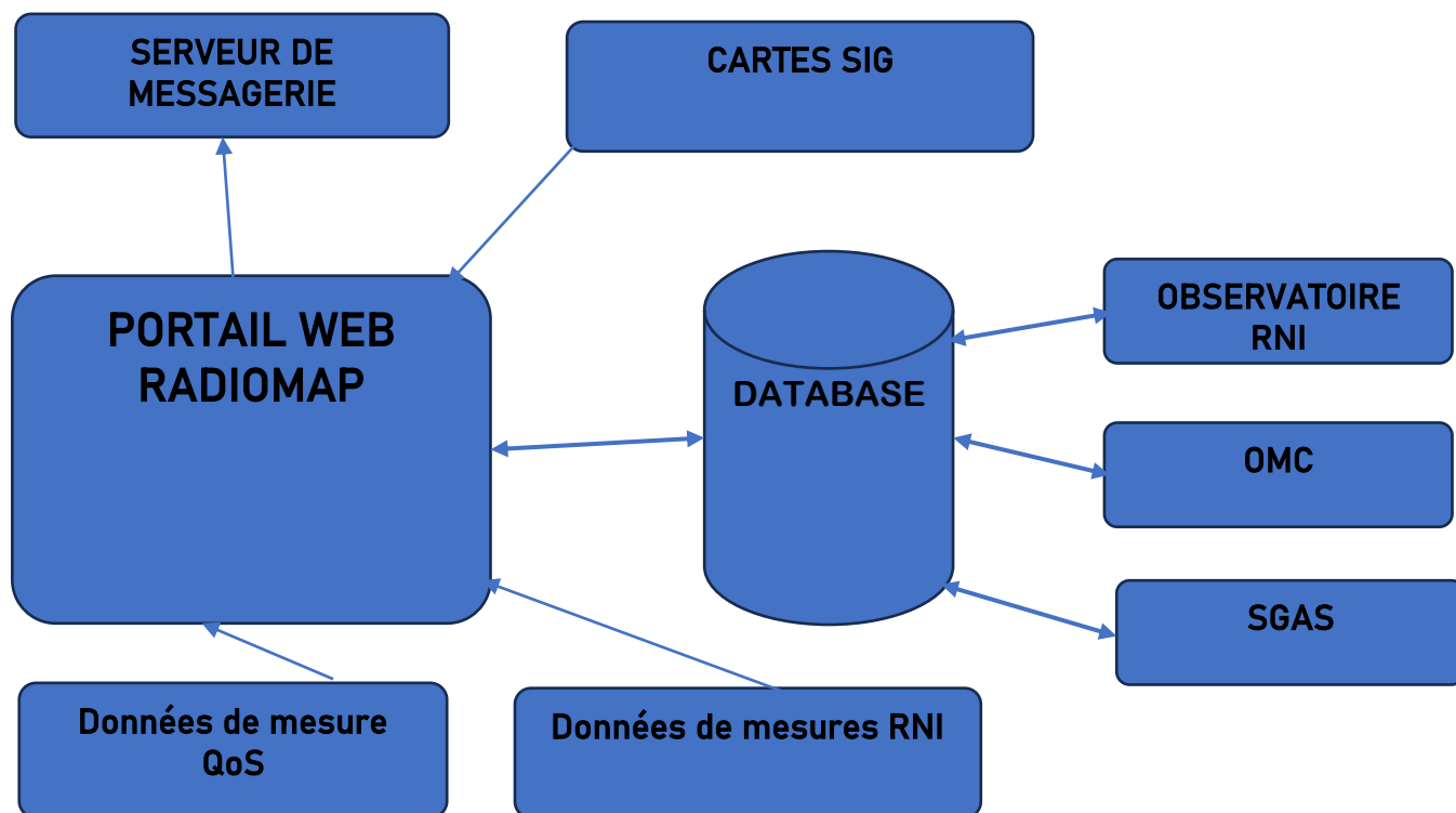
Figure 1 : Architecture de la plateforme « RadioMap »
